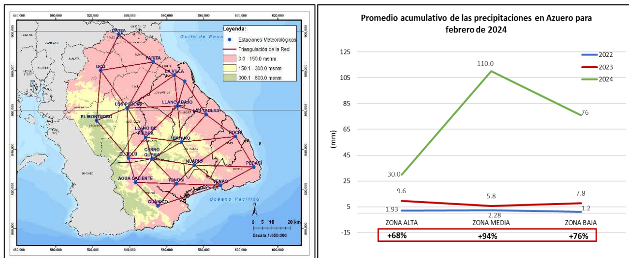
Figura 1. Promedio acumulado de las precipitaciones en tres zonas de Azuero durante febrero de 2024. Las zonas están determinadas por su elevación de la siguiente manera: Zona bajas de 0 a 150 msnm , Zonas medias de 151 a 300 msnm y Zonas altas de 301 a 600 msnm . mm=milímetros.
