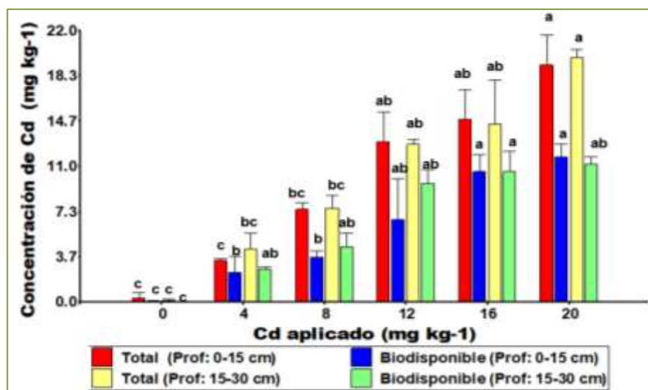
Figura 1. Concentraciones de Cd total y biodisponible en el suelo determinadas a dos profundidades del suelo (0 a 15 cm y 15 a 30 cm) con incrementos de dosis de Cd aplicadas al suelo.
